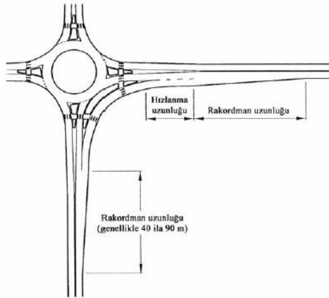
Şekil 2.55: Dönele kavşakta ilave sağ dönüş şeridi tasarımı
