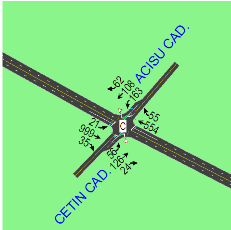
Şekil 7.104: Tavukçuyolu Caddesi&Acisu Caddesi&Çetin Caddesi kavşağı Syncro görünüşü
