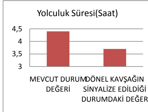
Şekil 7.24: Alemdağ Cd.- Adalet Sk.-30 Ağustos Sk. kavşağı yolculuk süresi grafiği
